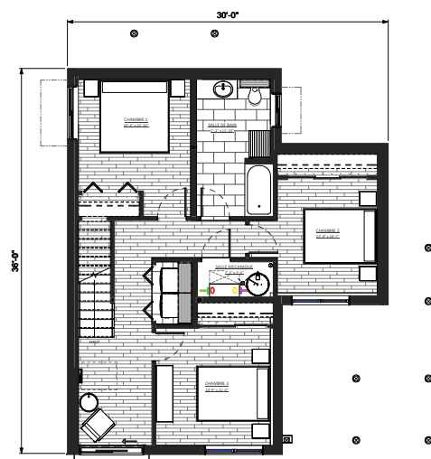
REZ-DE-JARDIN
