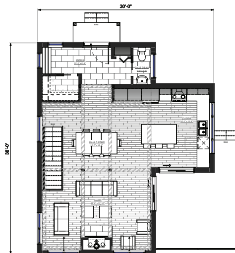
REZ-DE-CHAUSSÉE
